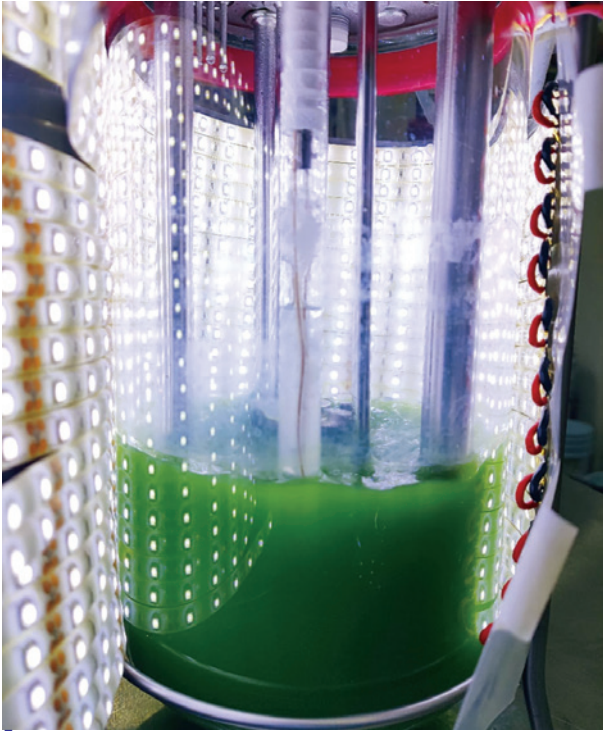
Figura 4. Captura de gases de efecto invernadero. Fuente: Sergio Revah.
