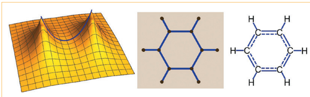
Figura 3. Caminos de enlace: en el extremo izquierdo, se muestra la trayectoria que une a dos carbonos adyacentes, la cual no tiene pendiente en la dirección que apunta al centro del benceno, por lo que no cae en dirección al centro. Fuente: elaboración propia.
