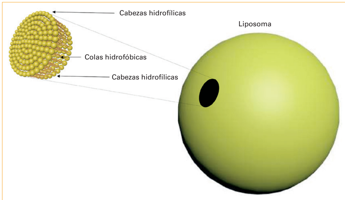
Figura 1. Liposoma y corte de la bicapa lipídica: tanto en el exterior como en el interior se encuentran las cabezas hidrofílicas; las colas hidrofóbicas están ubicadas entre las cabezas hidrofílicas. Estos dos sitios pueden ser utilizados para encapsular medicamentos. Fuente: elaboración propia.
