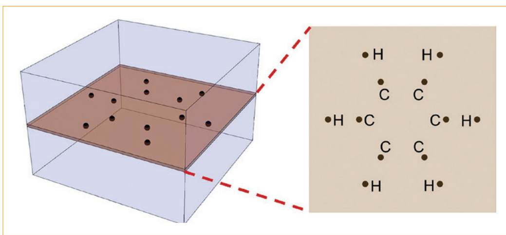
Figura 1. Para estudiar a la molécula de benceno, la colocamos en un espacio tridimensional. Luego, estudiaremos un segmento de todo el espacio, un corte que pasa por todos los núcleos de carbono e hidrógeno. Fuente: elaboración propia.
