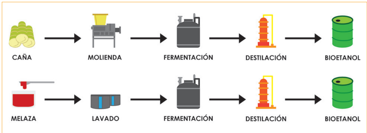
Figura 3. Proceso de producción de bioetanol a partir de: a) caña de azúcar; y b) melaza. Fuente: elaboración propia.
