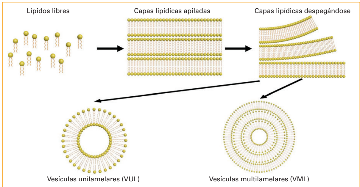
Figura 3. Los lípidos libres primero forman capas lipídicas apiladas en el fondo del recipiente; una vez que el solvente es removido, estas capas se despegan al ser rehidratadas y forman vesículas unilamelares o multilamelares. Fuente: elaboración propia.
