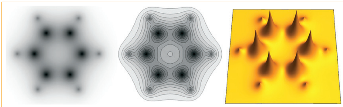
Figura 2. Densidad electrónica del benceno; en el extremo de la izquierda se muestra la densidad como un patrón de zonas oscuras (de alta densidad) y claras (de baja densidad). Para interpretarlo, se separa el mapa en regiones que tienen la misma densidad, como si fuera un mapa topográfico, mostrado al centro. Es posible representar la densidad en cada punto como una altura, y así obtener un paisaje tridimensional, como se aprecia en el extremo derecho. Fuente: elaboración propia.
