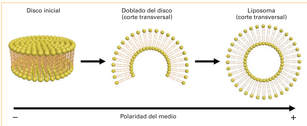
Figura 2. Los lípidos primero forman una doble capa lipídica en forma de disco; después se cierran en forma de esferas, debido al aumento de la polaridad del medio. Fuente: elaboración propia.
